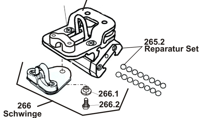
265 Kugellagertraveller kompl. ohne Schwinge
