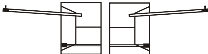
Ruderanlage kpl.(paar) ohne Ruderblatt Rudder housings cplt. without rudderblades
