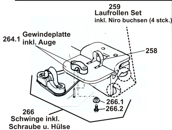
264 Rolltraveller kompl. ohne Schwinge
